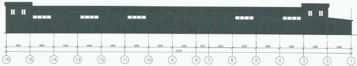
Фасад по оси Б
