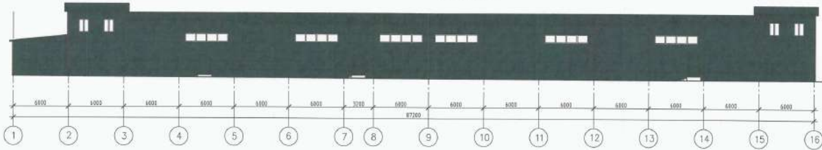
Фасад по оси А
