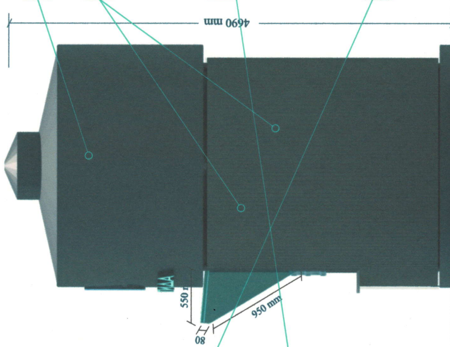
ВИД СПРАВА
