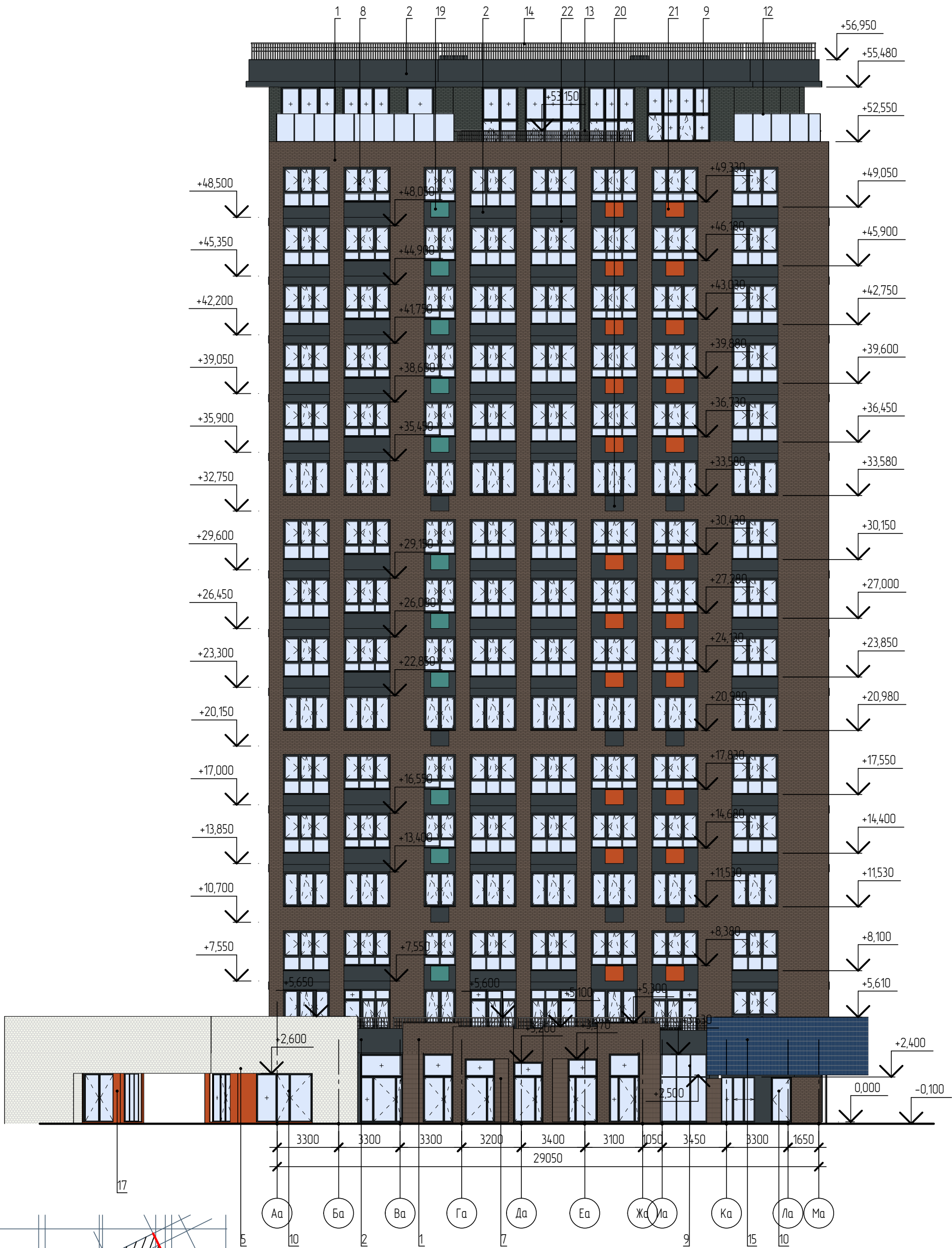
Фасад в осях Ас-Лс, М 1:200
