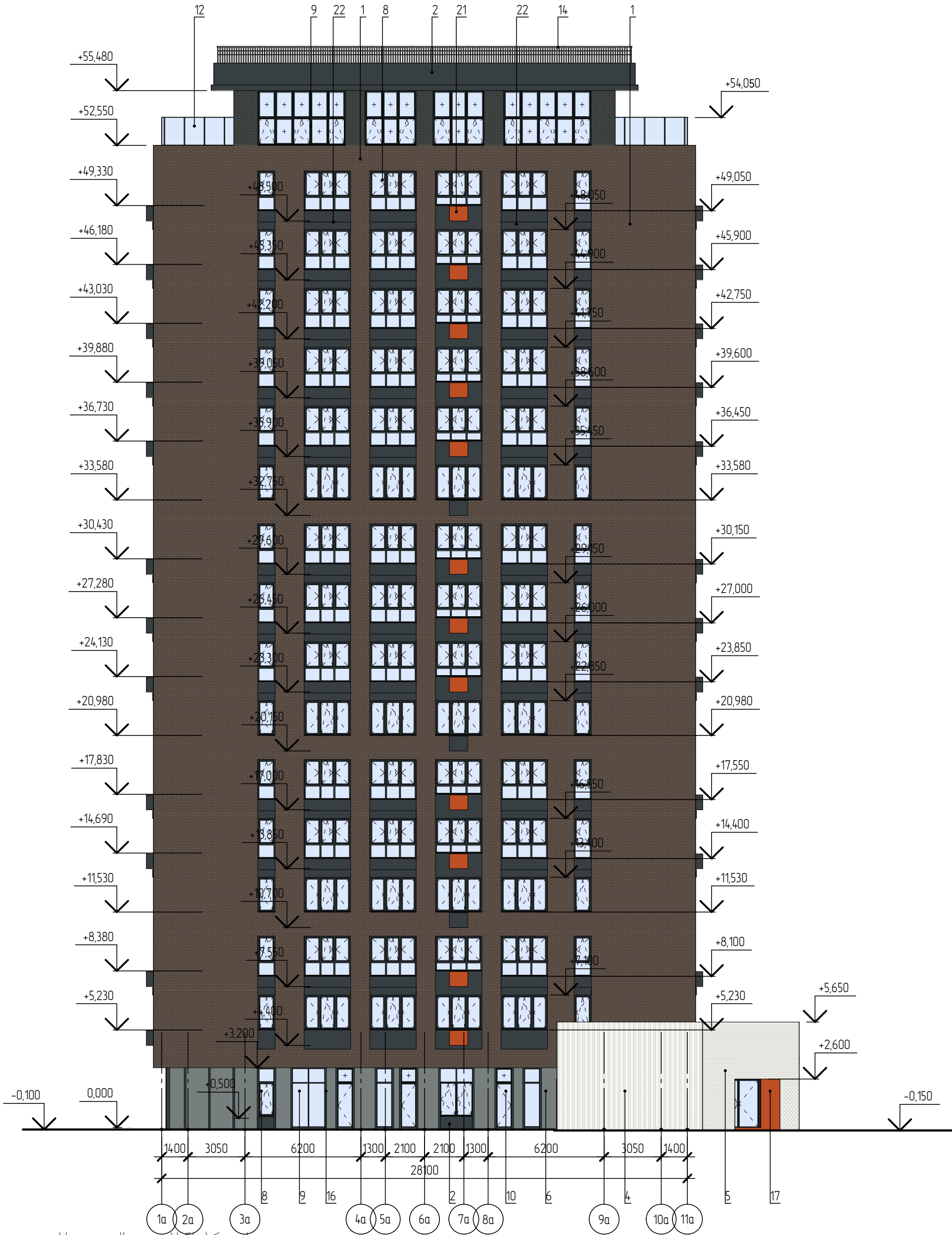
Фасад в осях 1с-9с, М 1:200
