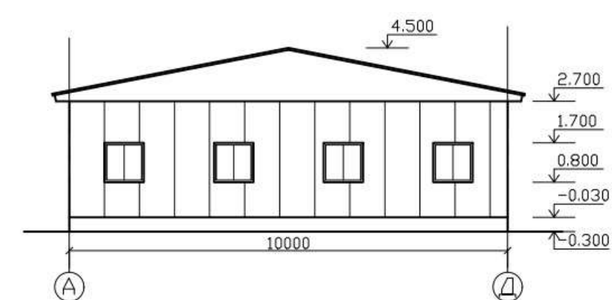
Фасад А-Д
