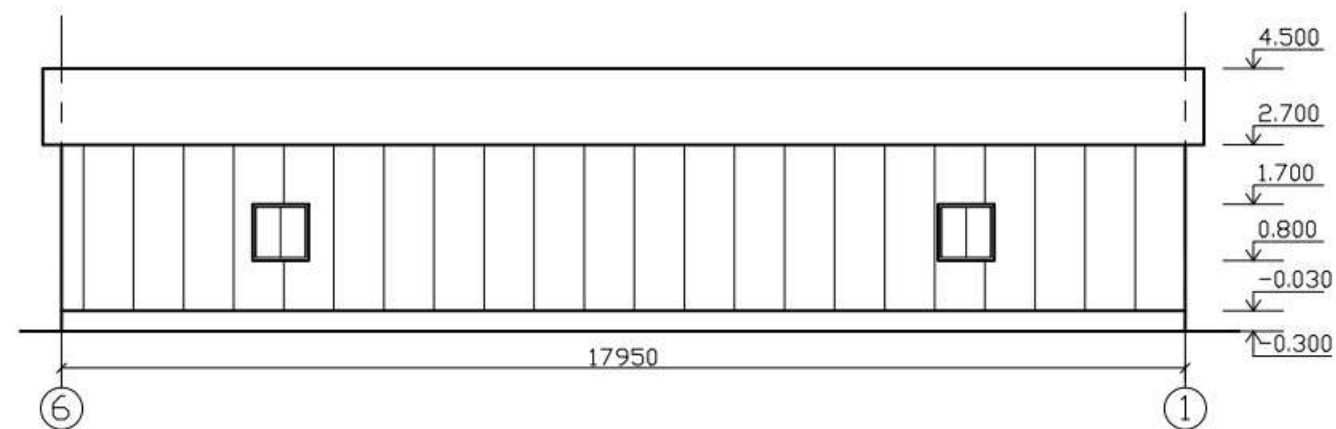
Фасад 6-1
