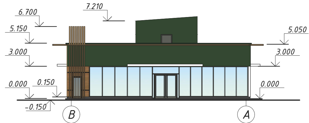
Фасад в осях В-А
