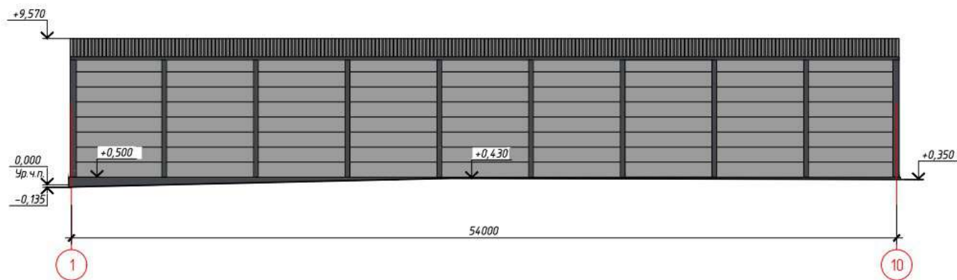
Фасад 1-10
