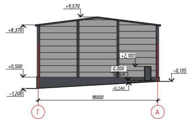
Фасад Г-А
