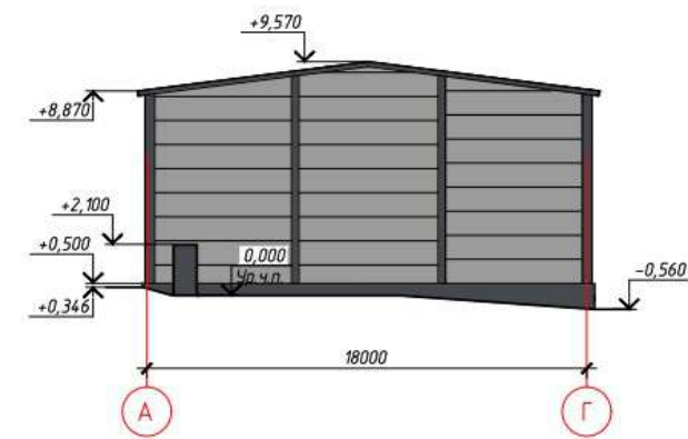
Фасад А-Г
