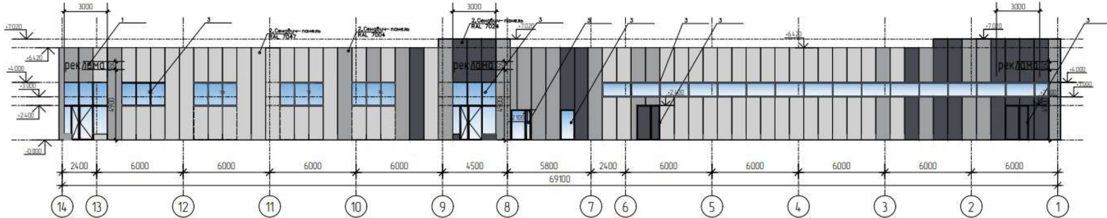
Фасад в осях 14-1
